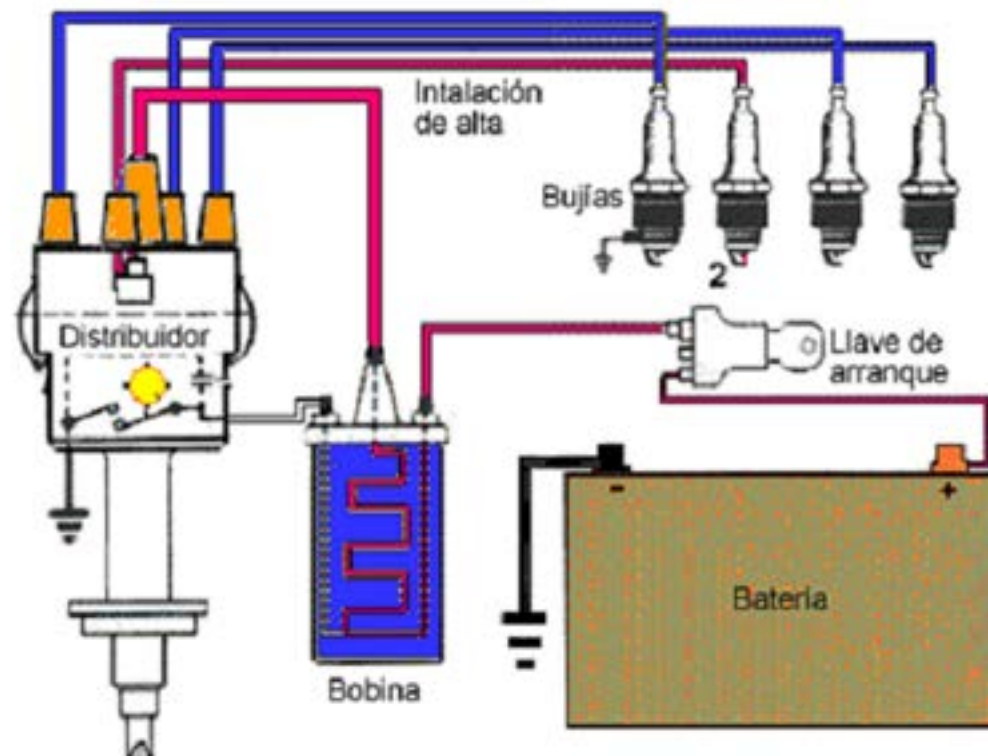
Proyecto, maqueta tipo interactiva perteneciente al diagrama general de un sistema de ignición.
