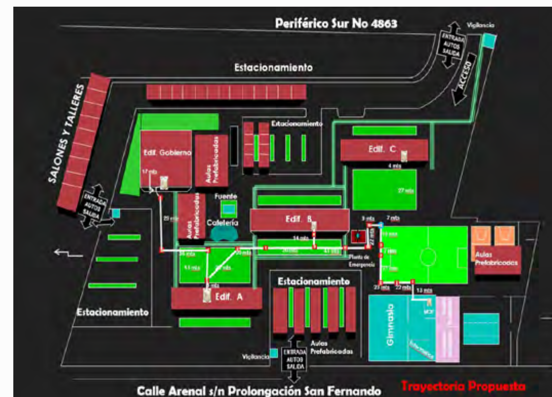
Croquis de Nueva Trayectoria de Fibra Óptica
