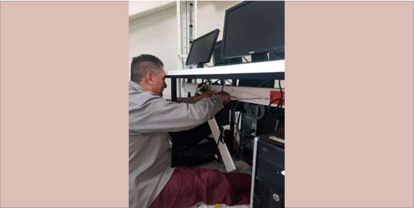
Instalación de contactos dobles polarizados en laboratorios de informática 1.
