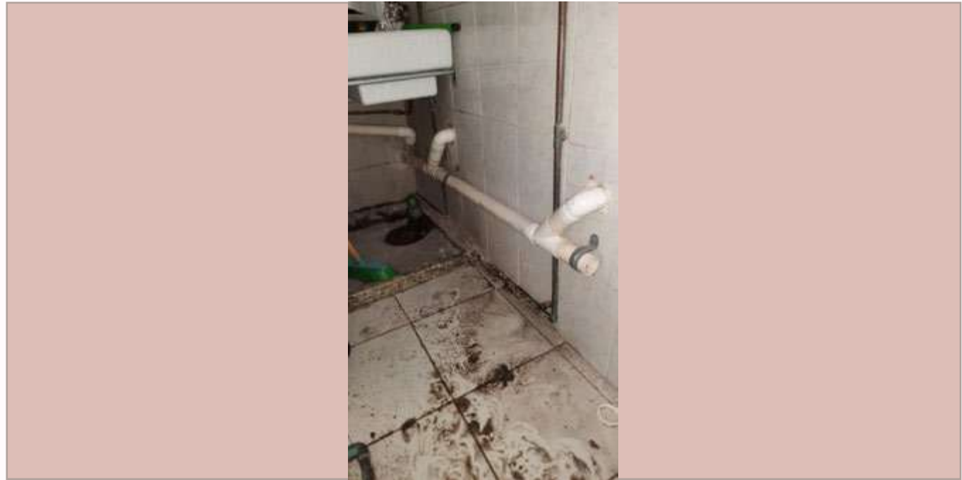
Reparación y desazolve de tubería de desagüe de lavabos en baño de hombres de planta alta en edificio de gobierno.
