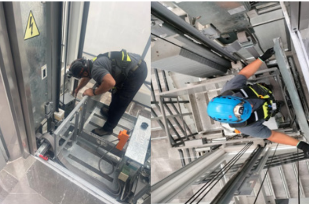
Mantenimiento preventivo y correctivo a elevadores del Instituto Nacional Politécnico.
